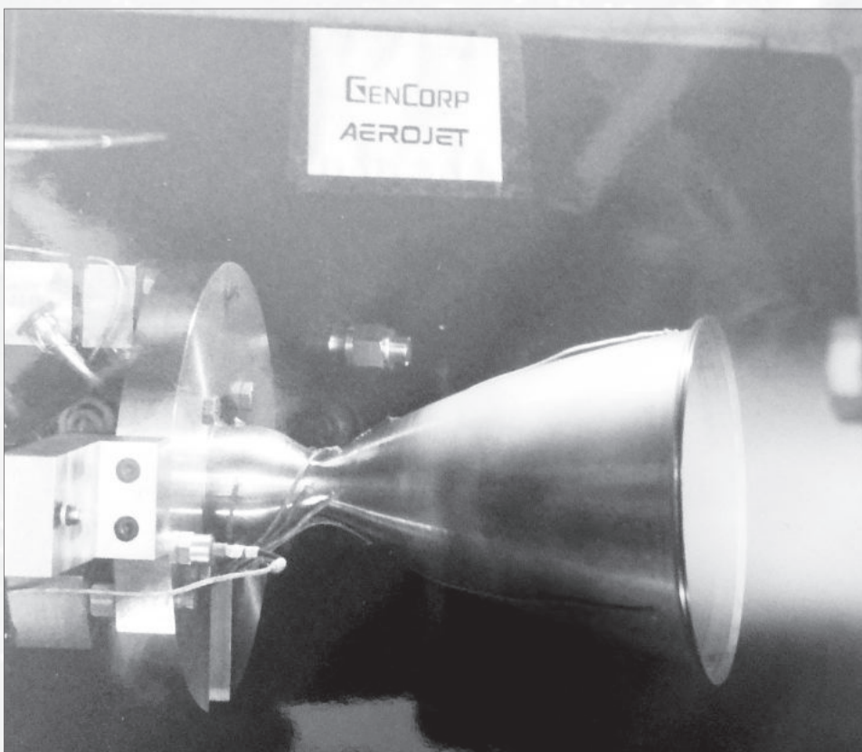
Двигатель тягой 40 кГ, разработки НИИМаш на стенде «Аэроджет» (США)
